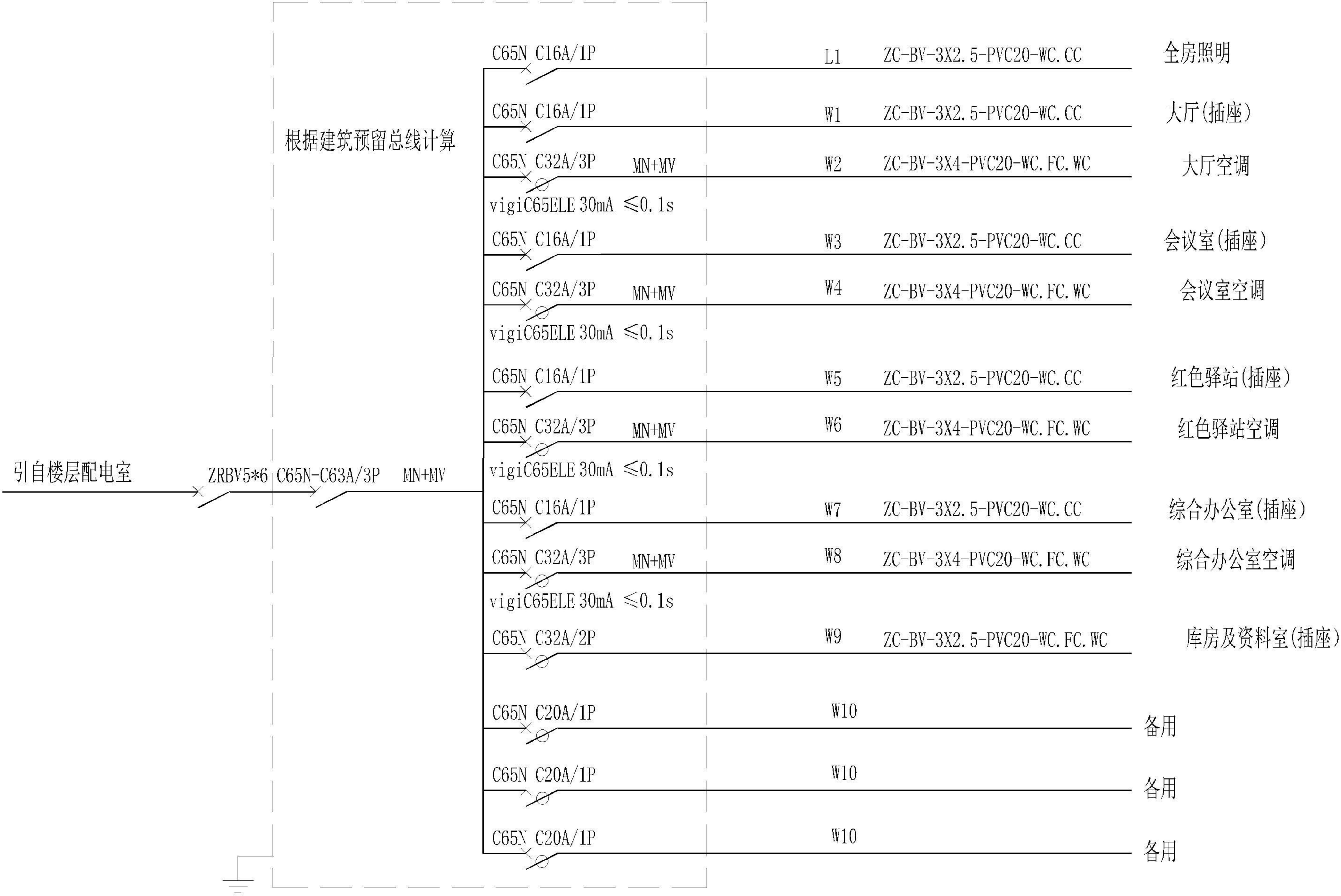
强电系统图
